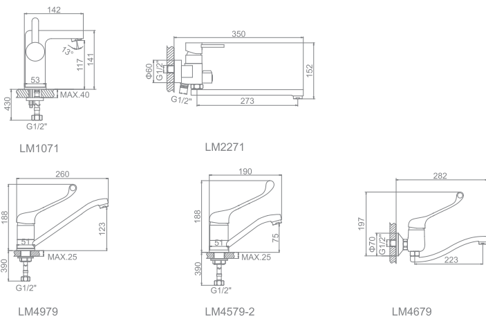
LM4579-2 Смеситель для кухни с коротким изливом
