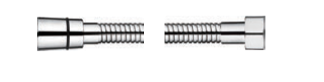
LM49-20 200см Хром Внутренняя труба из EPDM + оплётка из нерж. стали Латунная гайка Латунный конус Латунная торцевая втулка Защита от разрыва
