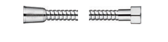
LM40-2 150см Внутренняя труба из PVC Нержавеющая гайка M22 (рус.) Конус из силумина M22 (рус.) Латунная торцевая втулка
