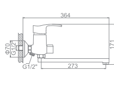
LM4564 Смеситель для кухни с коротким изливом
