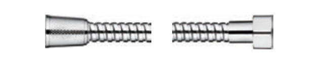
LM40 150см Внутренняя труба из PVC Нержавеющая гайка Конус из силумина Латунная торцевая втулка
