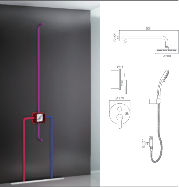
LM2403-2 Ø 40 Душевая система (встраиваемая) со смесителем и тропическим душем
