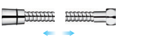
LM48 150-220см Хром Внутренняя труба из PVC Латунная гайка Конус из силумина Латунная торцевая втулка Растягивающийся от 150 до 220см
