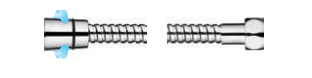
LM42 150см Хром Внутренняя труба из PVC Латунная гайка Латунный конус Латунная торцевая втулка Свободное вращение на 360°, защита от скручивания
