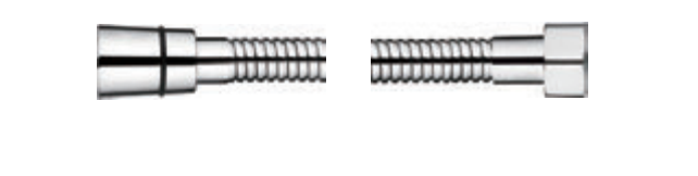
LM49-17 170см Хром Внутренняя труба из EPDM + оплётка из нерж. стали Латунная гайка Латунный конус Латунная торцевая втулка Защита от разрыва
