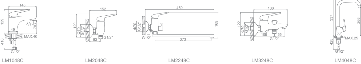
LM3248C Смеситель для ванны с коротким изливом. Дивертор в корпусе
