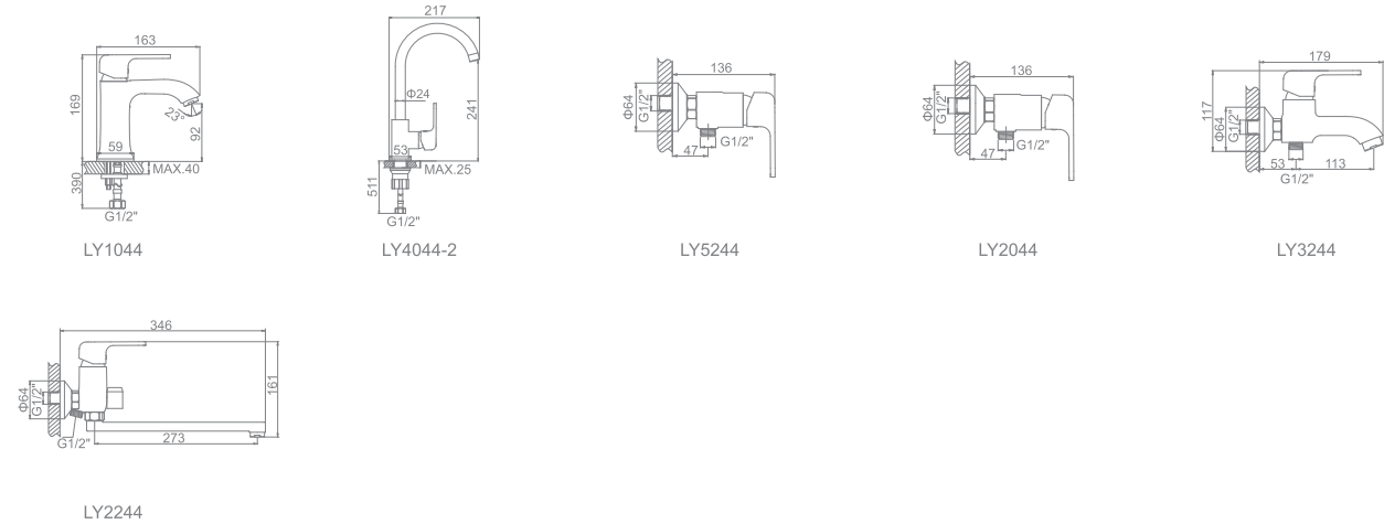
LY2244 Излив :L30F Смеситель для ванны с длинным изливом 300мм. Дивертор в корпусе
