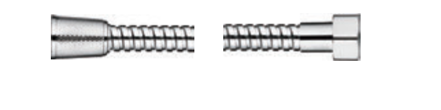
LM40-1 150см Внутренняя труба из PVC Нержавеющая гайка M22 (рус.) Конус из силумина 1/2 (имп.) Латунная торцевая втулка
