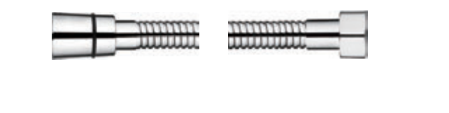
LM49 150см Хром Внутренняя труба из EPDM + оплётка из нерж. стали Латунная гайка Латунный конус Латунная торцевая втулка Защита от разрыва
